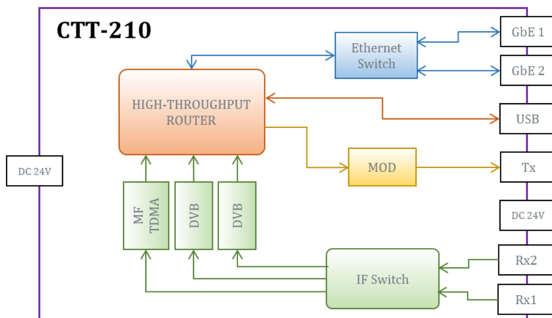
Рисунок 5. Структурная схема маршрутизатора СТТ-200
