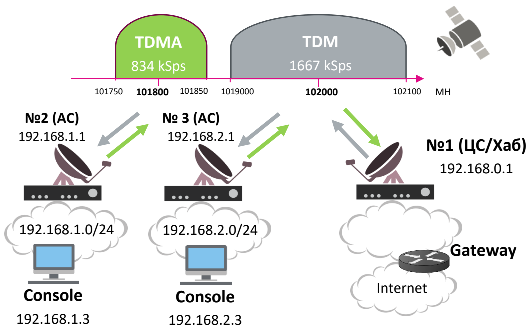
Рисунок 2. Пример схемы организации VSAT-сети
