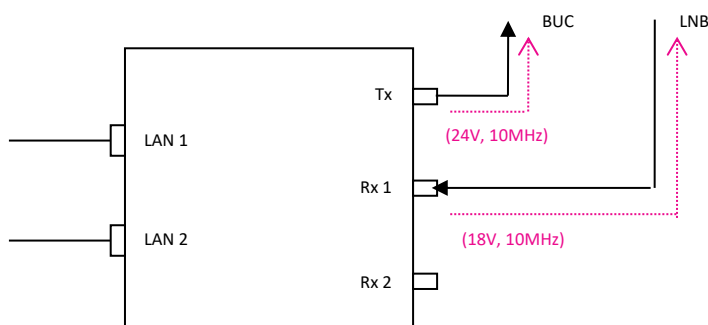
Рисунок 8. Схема стандартного подключения маршрутизатора СТТ-200
